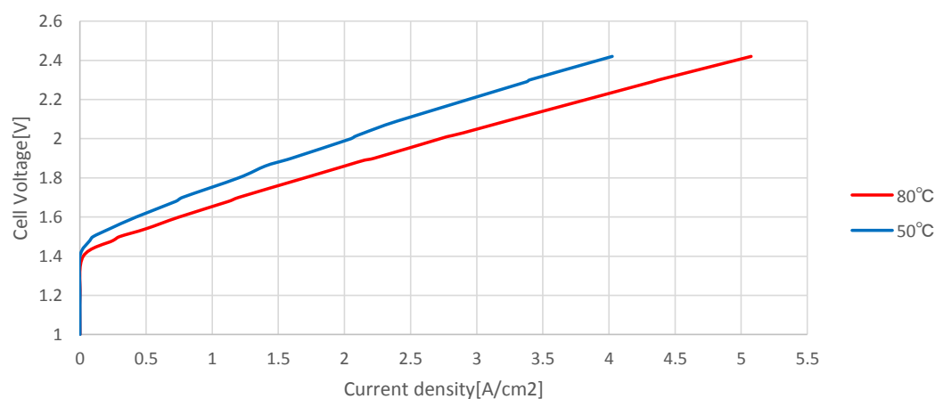
<参考値>I-Vカーブ
